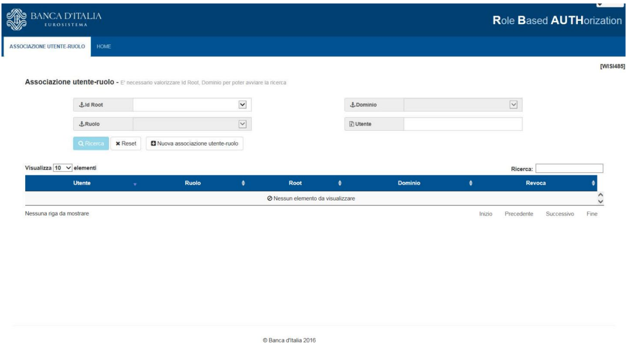
Figura 27 – Associazione utente-ruolo
